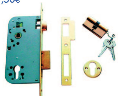
Ref. A005328 CERRADURA EMBUTIR SERIE 203050HL TESA
